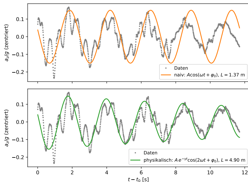
Abbildung 2: Oben: das naive, ungedämpfte Ein-Frequenz-Modell aus Aufgabe 3. Unten: ein von Hand nachgebessertes Modell mit doppelter Frequenz 2\omega und Dämpfung e^{-\gamma t} – deutlich zu erkennen, wie die abklingende Hüllkurve die Daten jetzt über das ganze Fenster hinweg viel besser trifft.
