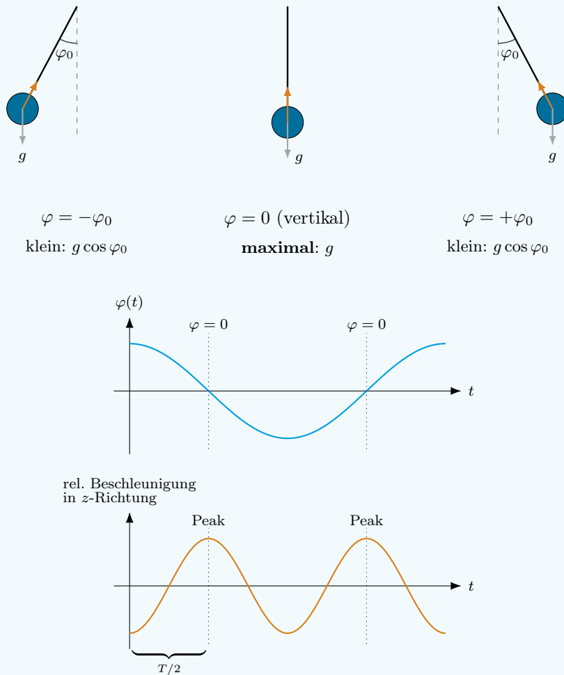
Abbildung 1: Oben: das Pendel an den beiden Umkehrpunkten und im Nulldurchgang, jeweils mit dem Schwerkraftvektor g (grau, immer senkrecht nach unten mit gleicher Stärke) und der Komponente entlang der Schnur, die zur Aufhängung zeigt und die das Handy als Beschleunigung misst (orange). Diese Komponente muss zur Aufhängung hin zeigen – sie hält den Pendelkörper ja auf seiner Kreisbahn, statt ihn einfach nach unten fallen zu lassen. Ihre Stärke ist g \cos \varphi : am Umkehrpunkt am kleinsten, im Nulldurchgang (vertikal) am größten. Unten: Da \varphi(t) zweimal pro Periode T durch \varphi = 0 läuft, hat das gemessene Signal \propto g \cos \varphi(t) auch zwei Maxima pro Periode – die doppelte Frequenz 2\omega .
