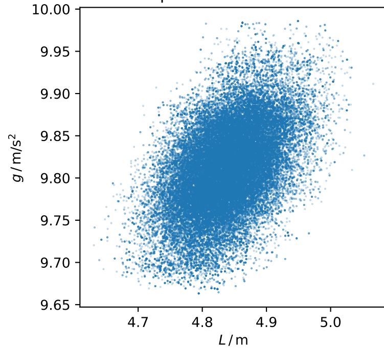
Samples nach dem burn-in
